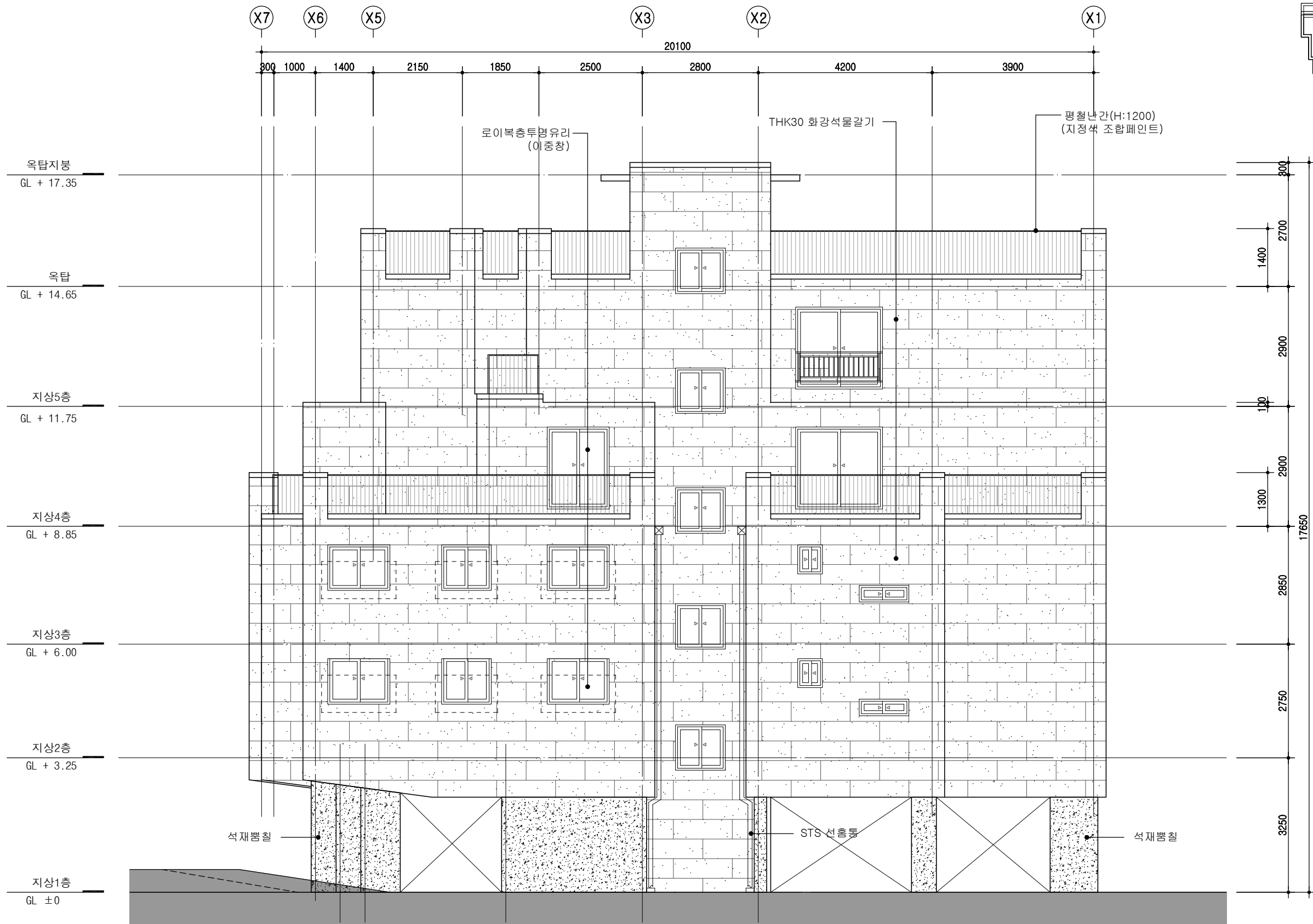
서 측 면 도 SCALE: 1 / 100
