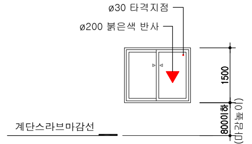
소방관 진입창
