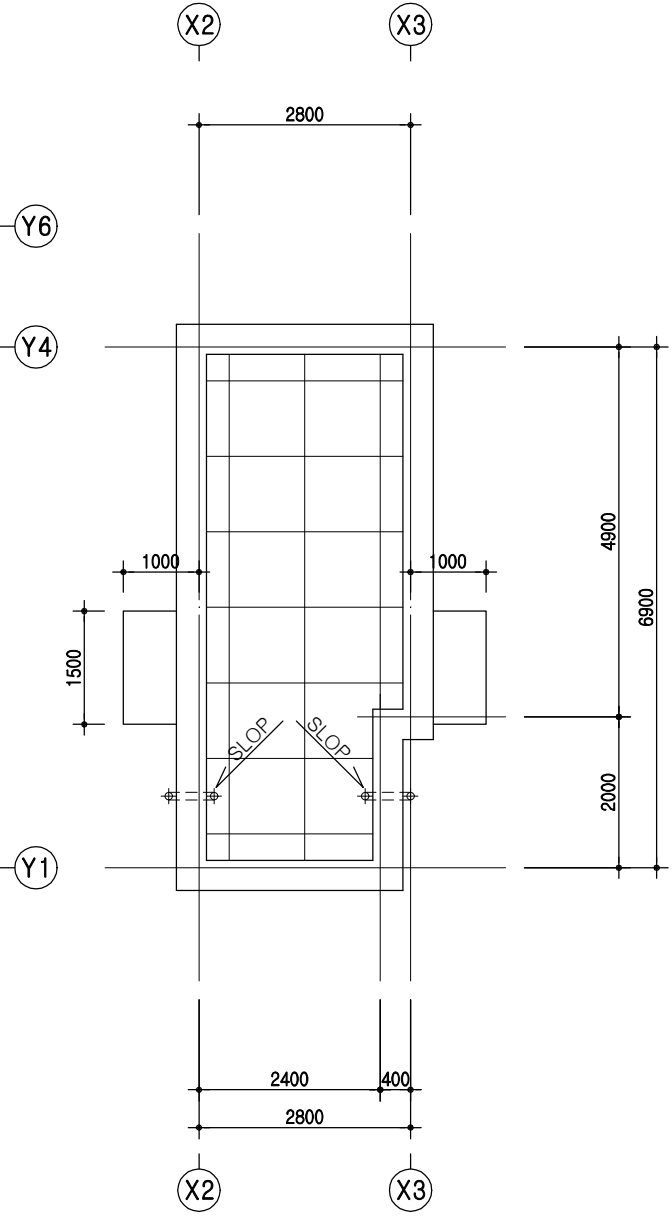
옥탑지붕 평면도 SCALE: 1 / 100
