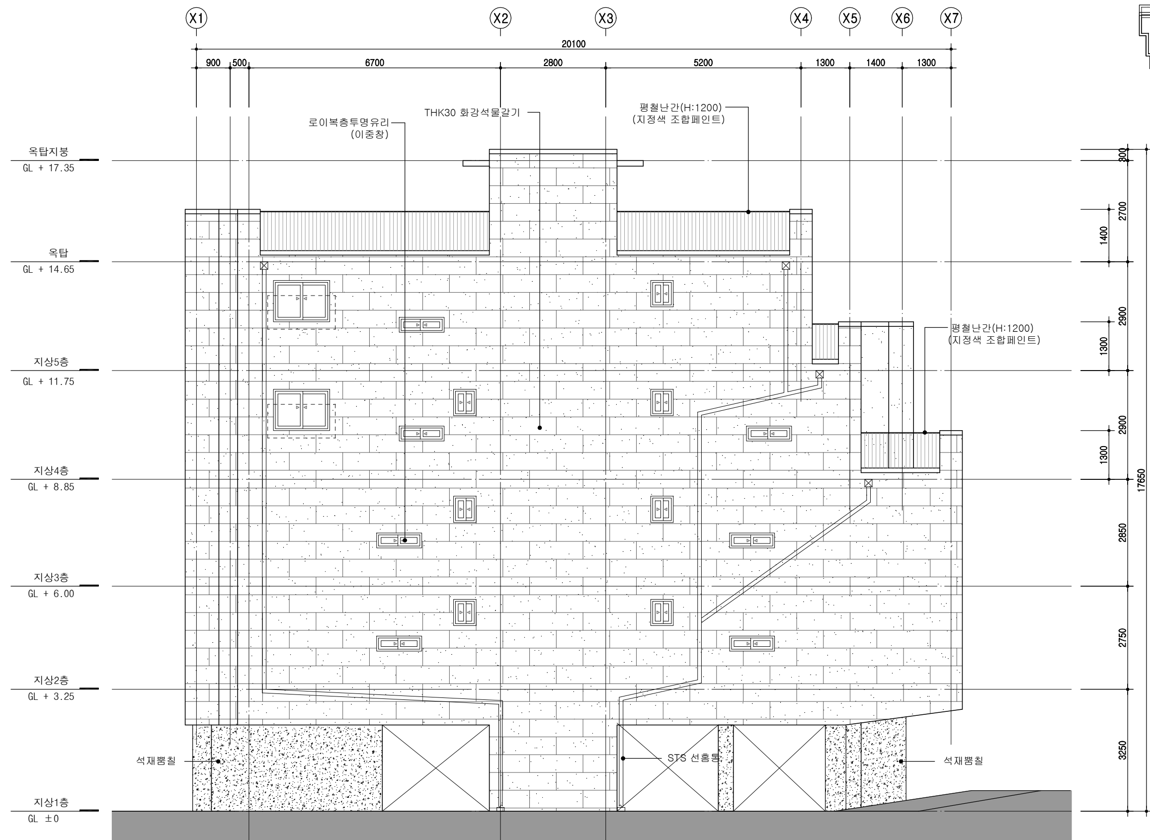
동측면도 SCALE: 1 / 100
