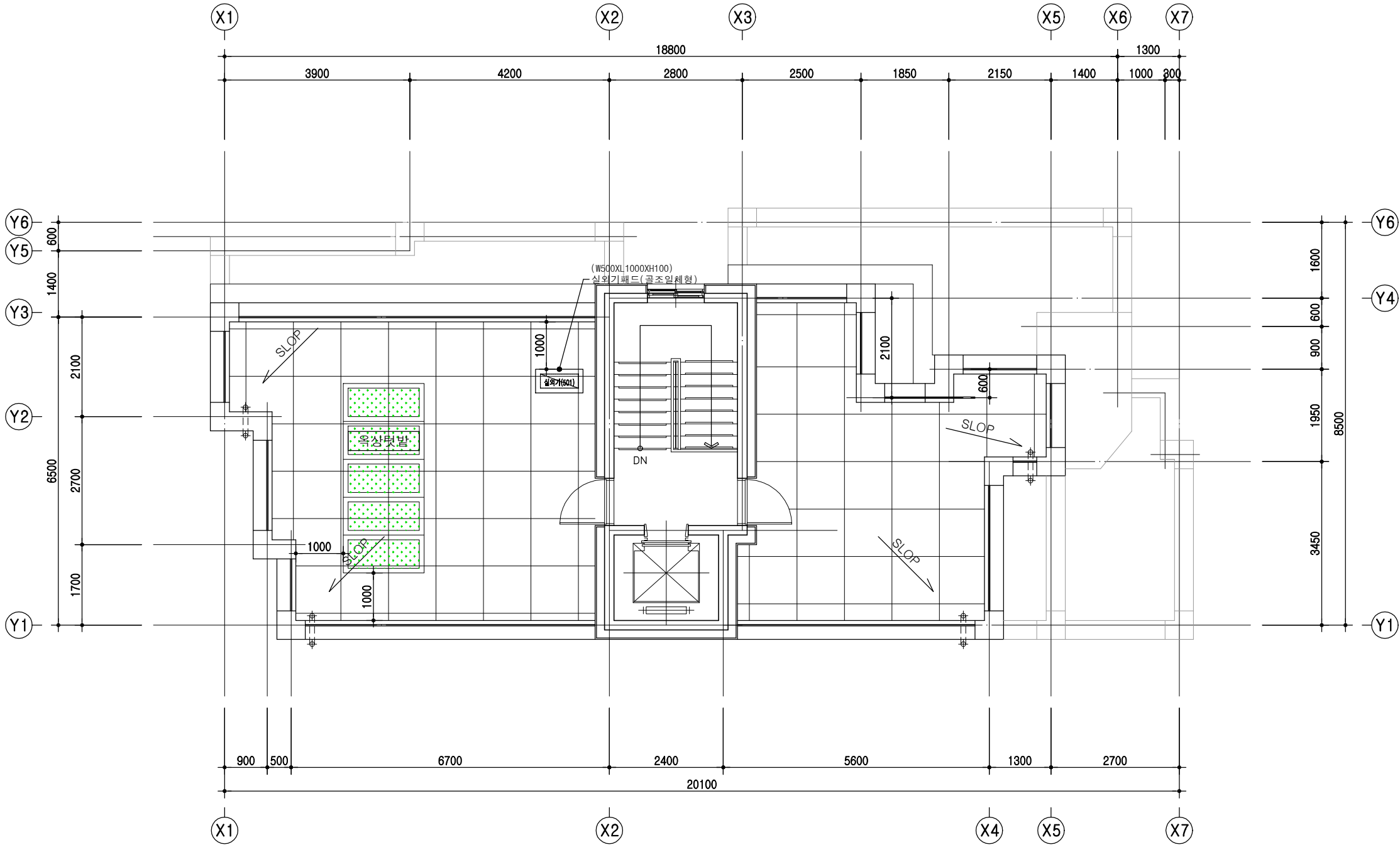
지붕층 평면도 SCALE: 1 / 100
