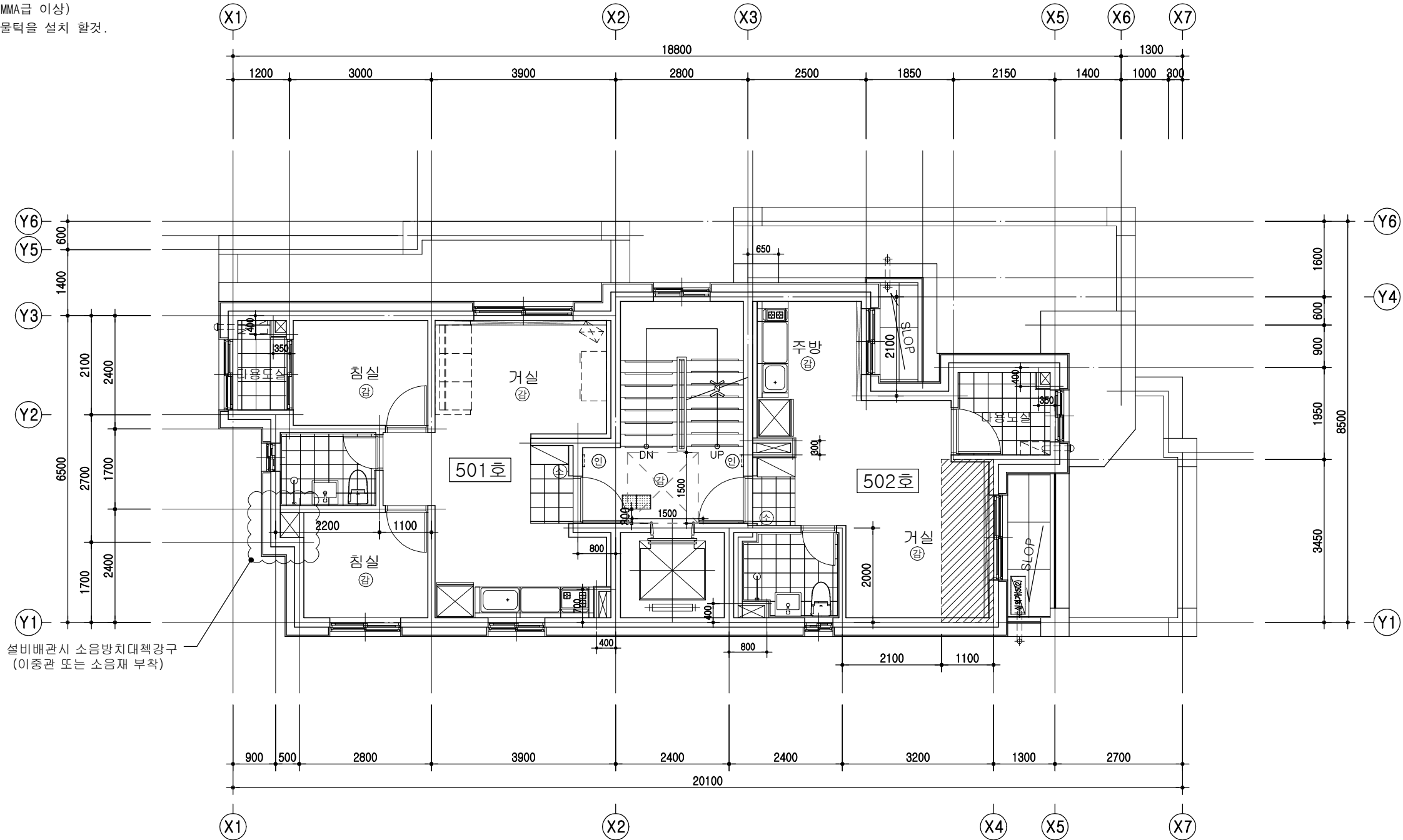
5 층 평 면 도 SCALE: 1 / 100
